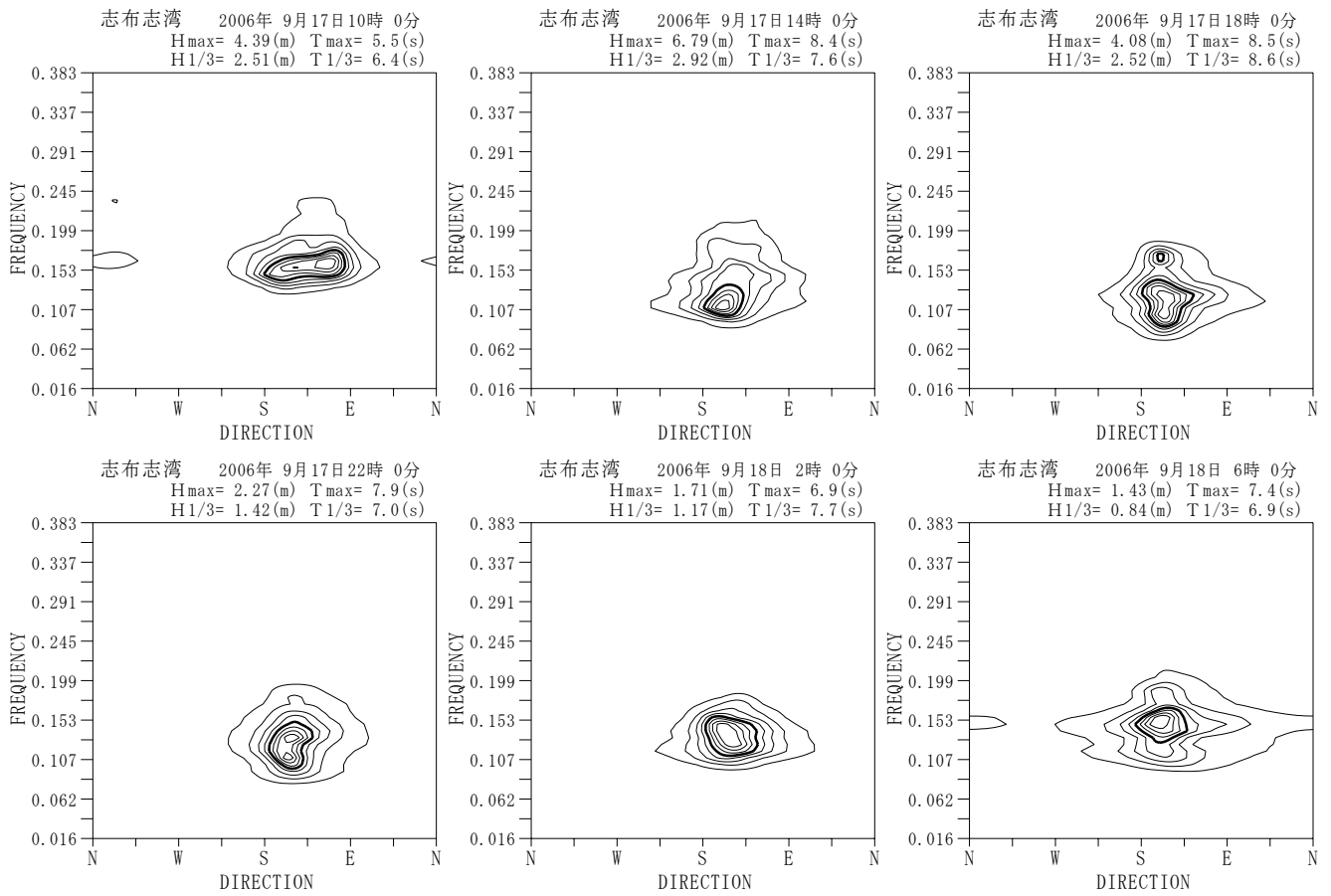
付図-A.5.57 志布志湾 代表的な高波期間中の方向スペクトル
