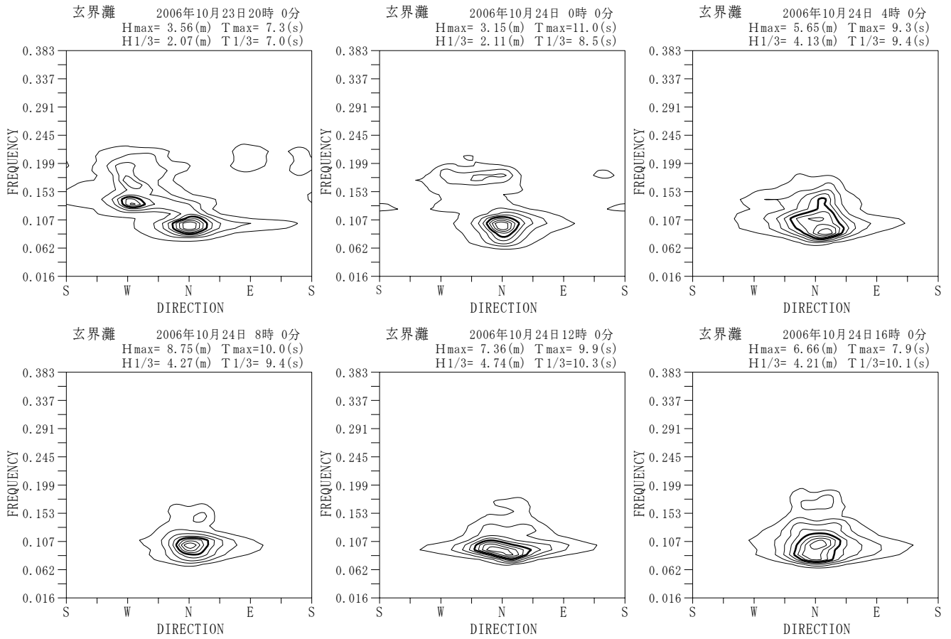
付図-A. 5. 22 玄界灘 代表的な高波期間中の方向スペクトル
