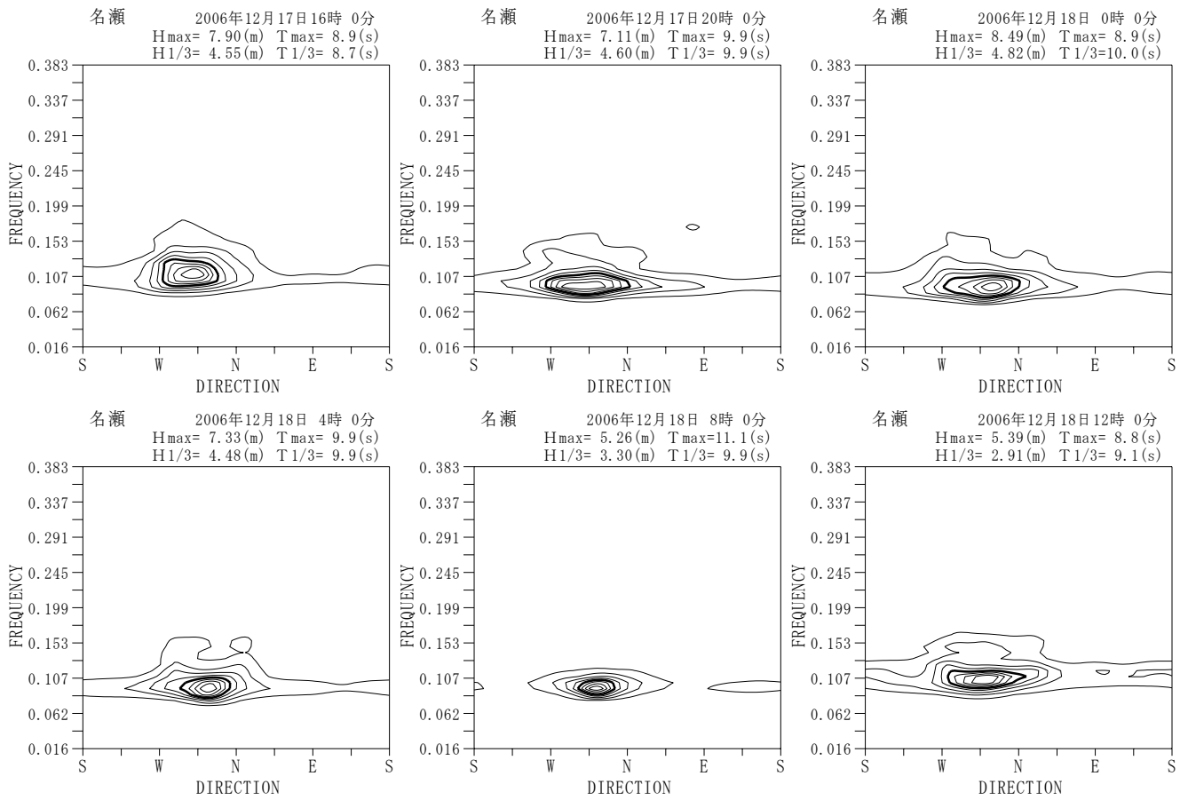
付図-A. 5. 25 名瀬 代表的な高波期間中の方向スペクトル
