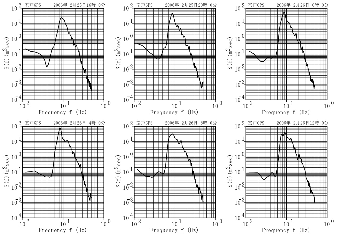
付図-A.5.51 室戸GPS 代表的な高波期間中のスペクトル
