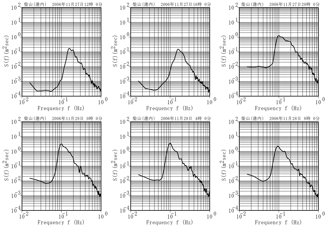
付図-A.5.17 柴山(港内) 代表的な高波期間中のスペクトル
