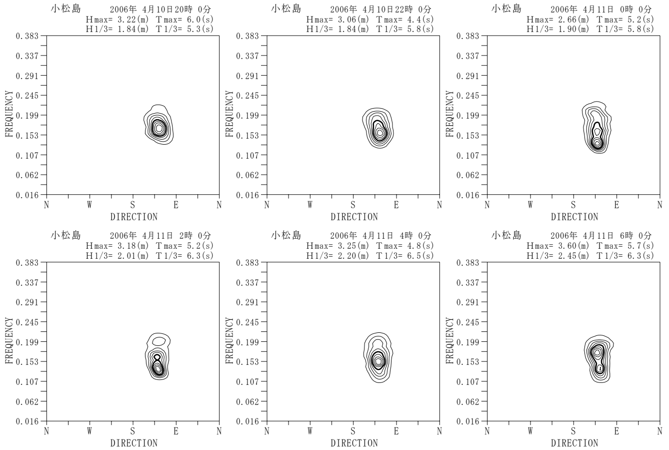
付図-A. 5. 50 小松島 代表的な高波期間中の方向スペクトル
