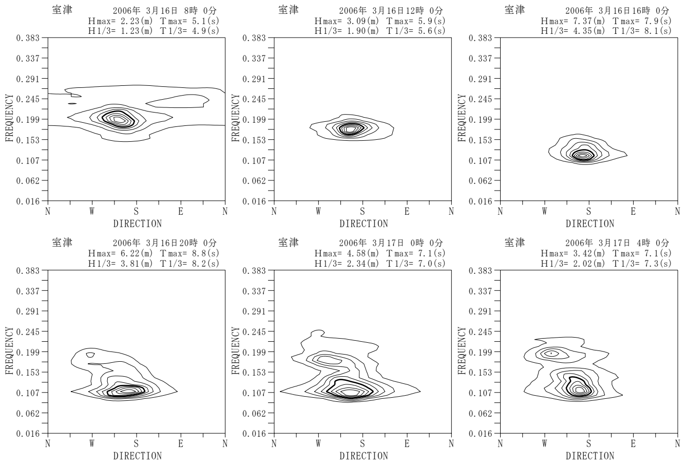
付図-A. 5.52 室津 代表的な高波期間中の方向スペクトル
