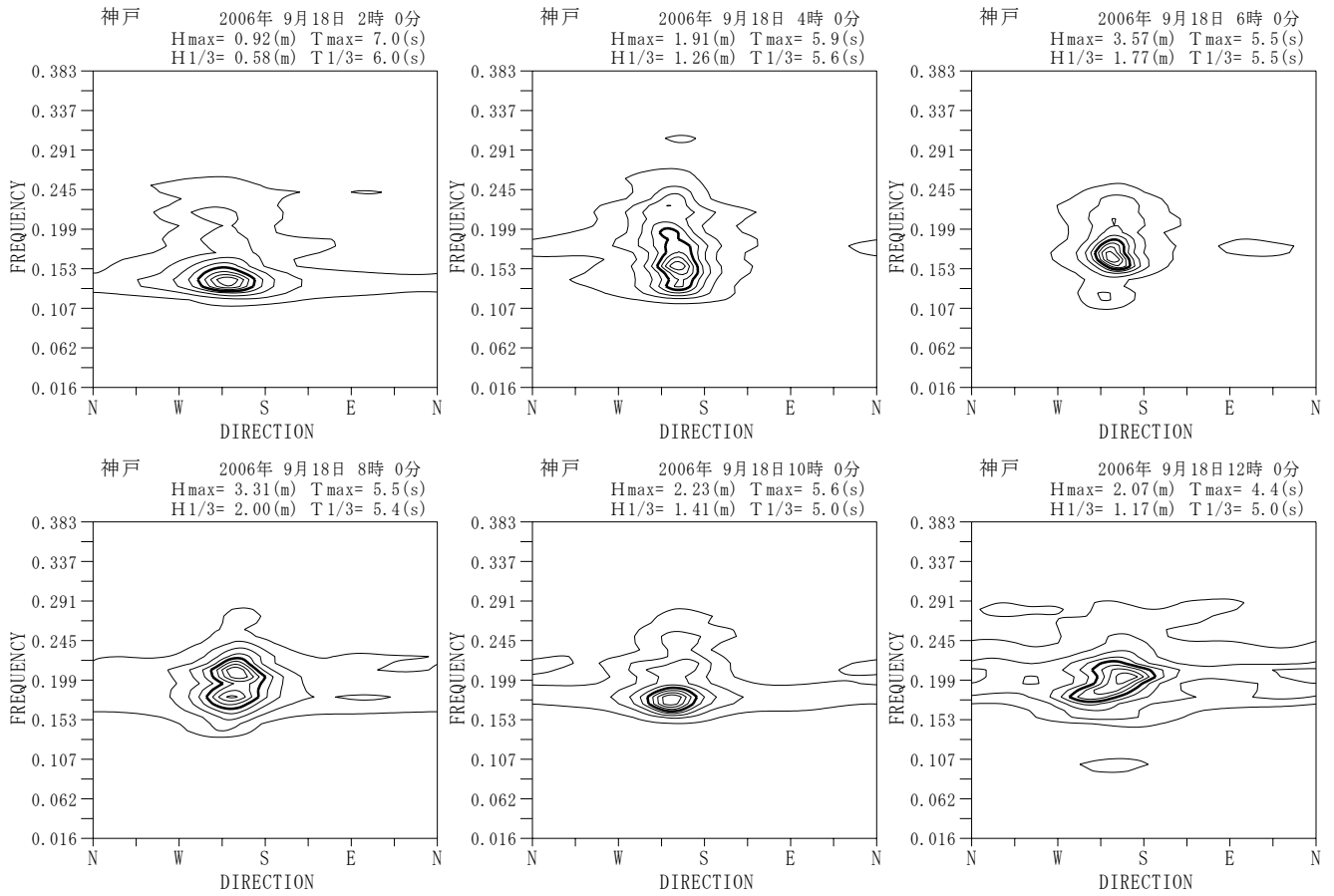
付図-A. 5. 49 神戸 代表的な高波期間中の方向スペクトル
