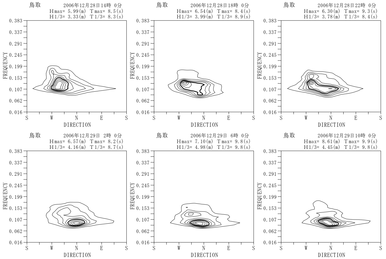
付図-A. 5. 18 鳥取 代表的な高波期間中の方向スペクトル
