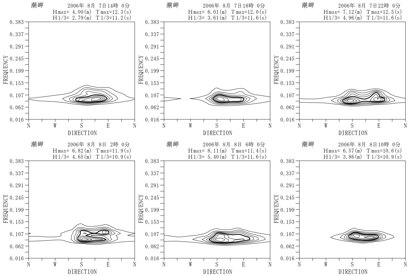
付図-A. 5. 48 潮岬 代表的な高波期間中の方向スペクトル
