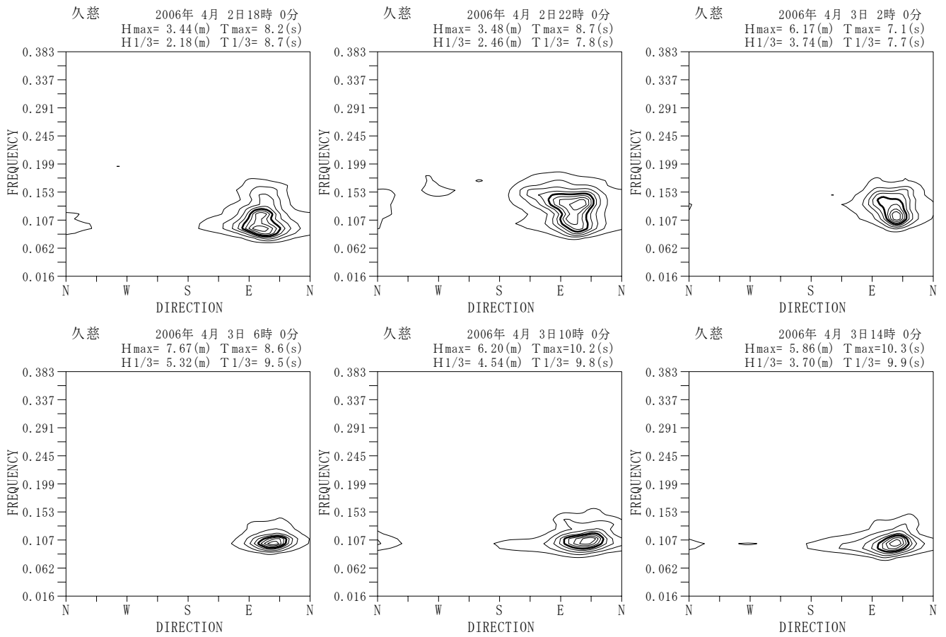
付図-A. 5.33 久慈 代表的な高波期間中の方向スペクトル
