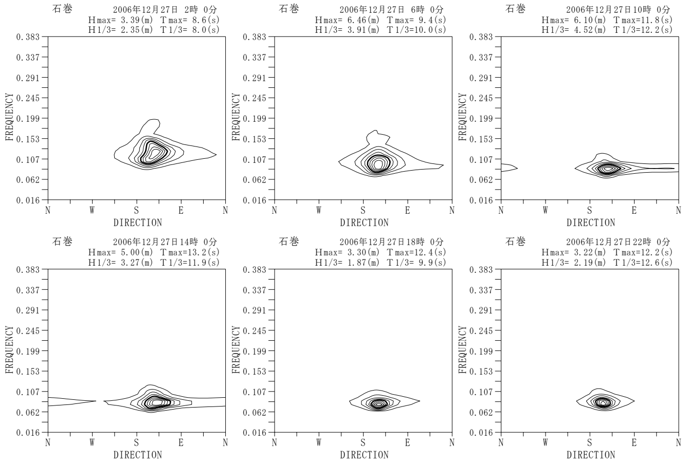
付図-A. 5. 35 石巻 代表的な高波期間中の方向スペクトル
