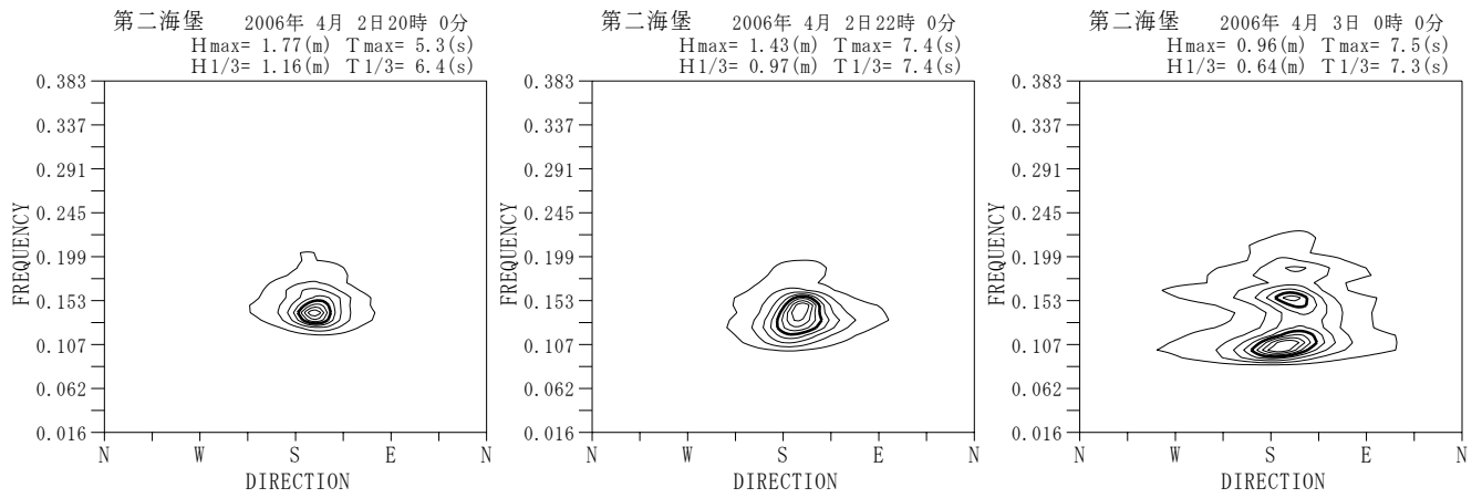
付図-A.5.41 第二海堡 代表的な高波期間中の方向スペクトル
