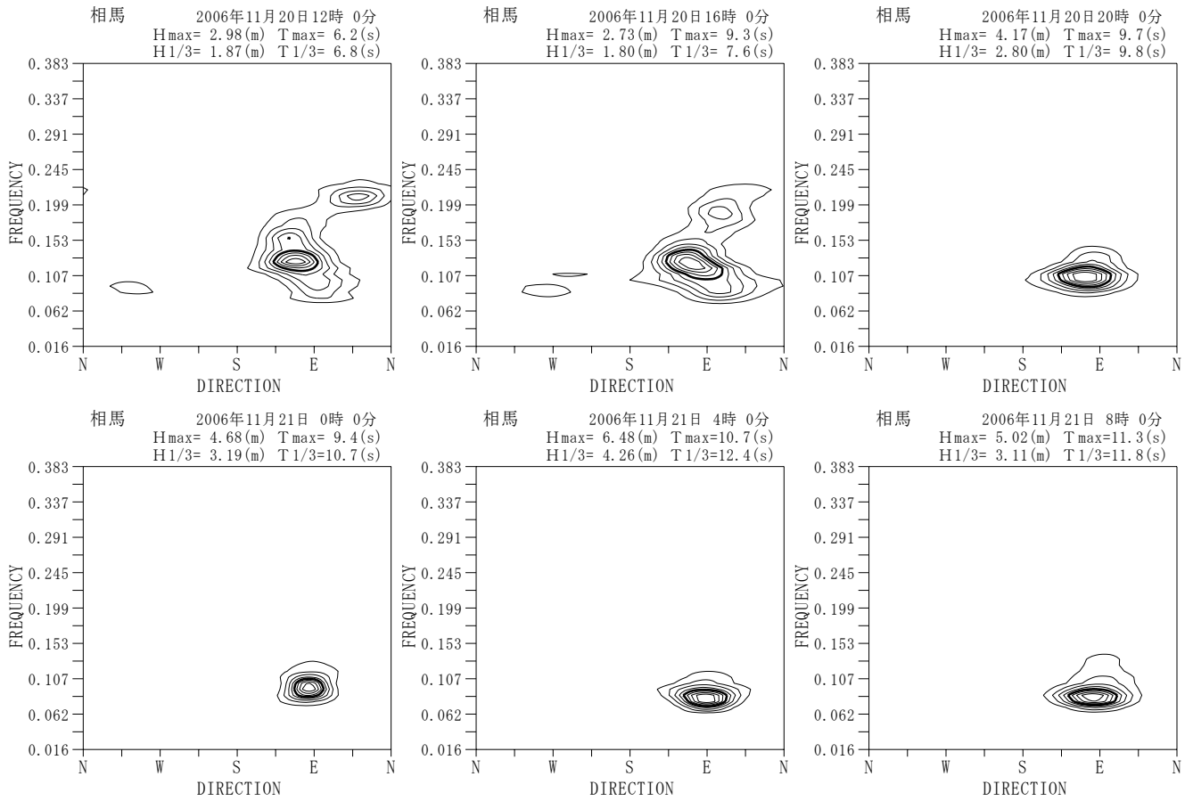
付図-A. 5. 37 相馬 代表的な高波期間中の方向スペクトル
