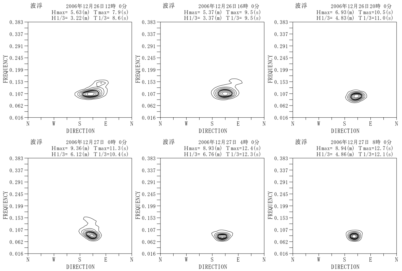
付図-A. 5. 43 波浮 代表的な高波期間中の方向スペクトル
