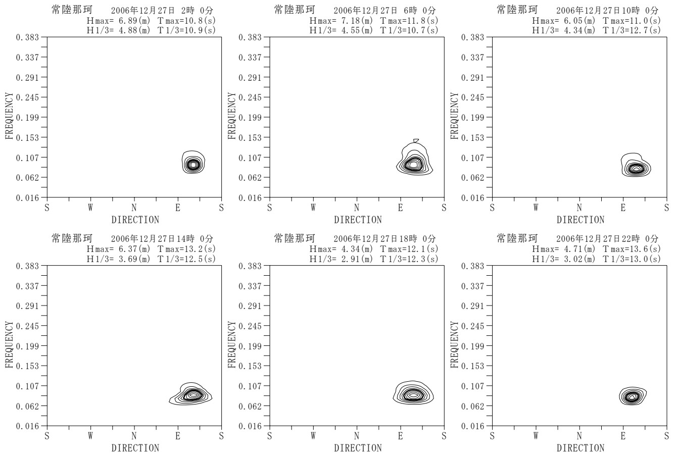
付図-A.5.39 常陸那珂 代表的な高波期間中の方向スペクトル
