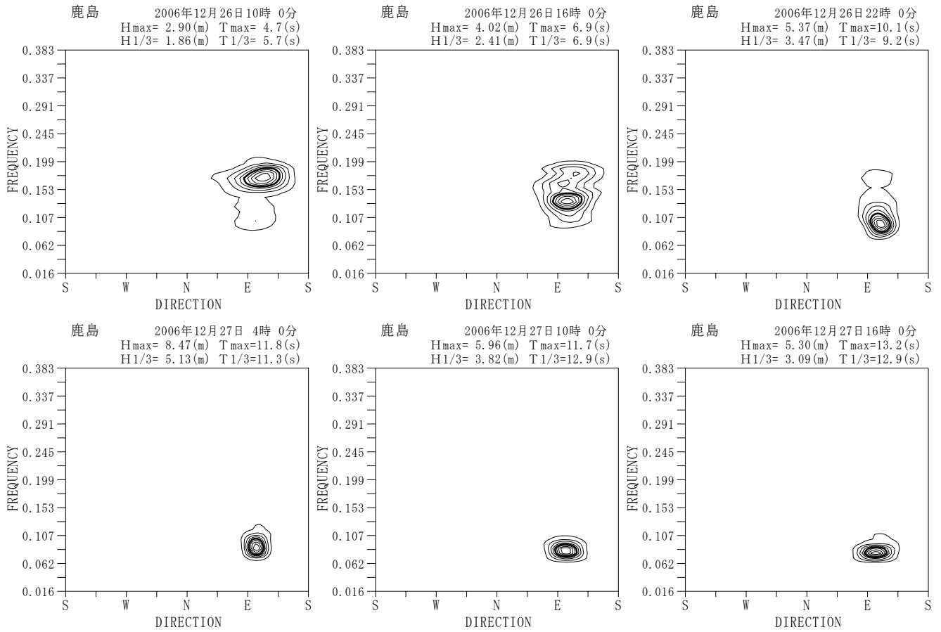
付図-A. 5. 40 鹿島 代表的な高波期間中の方向スペクトル
