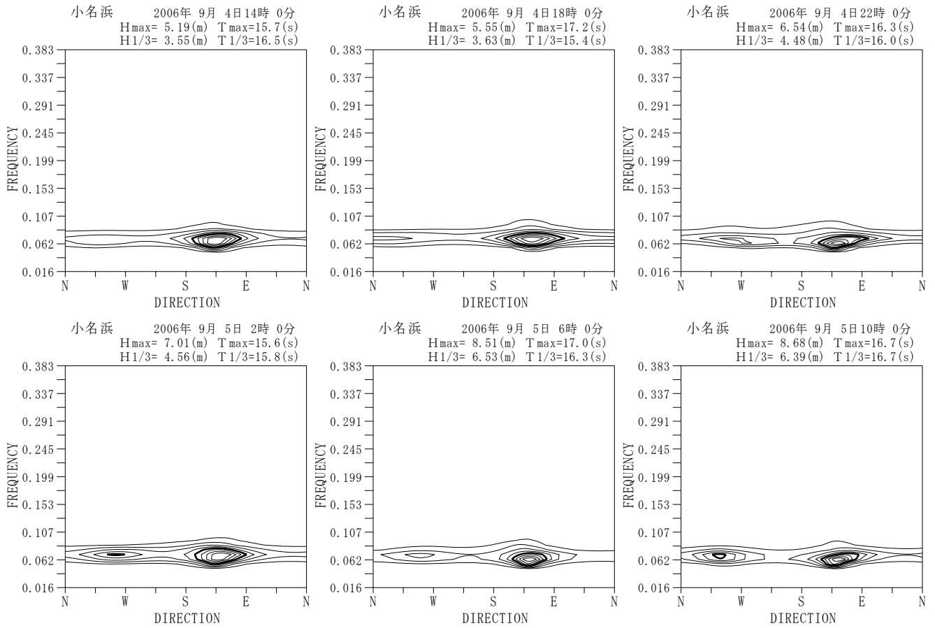
付図-A. 5. 38 小名浜 代表的な高波期間中の方向スペクトル
