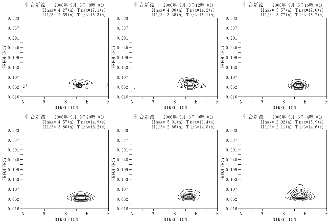
付図-A.5.36 仙台新港 代表的な高波期間中の方向スペクトル
