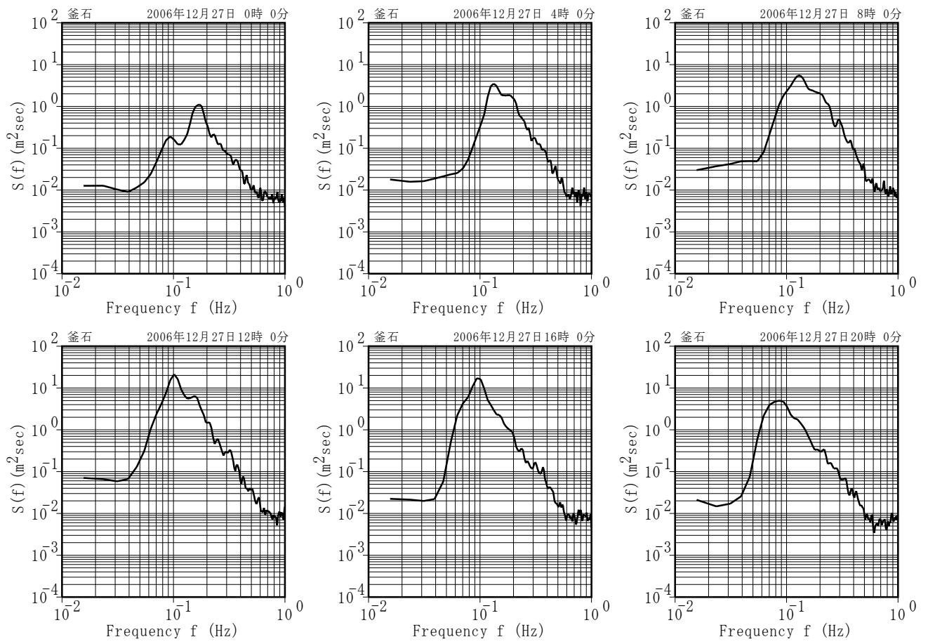
付図-A.5.34 釜石 代表的な高波期間中のスペクトル
