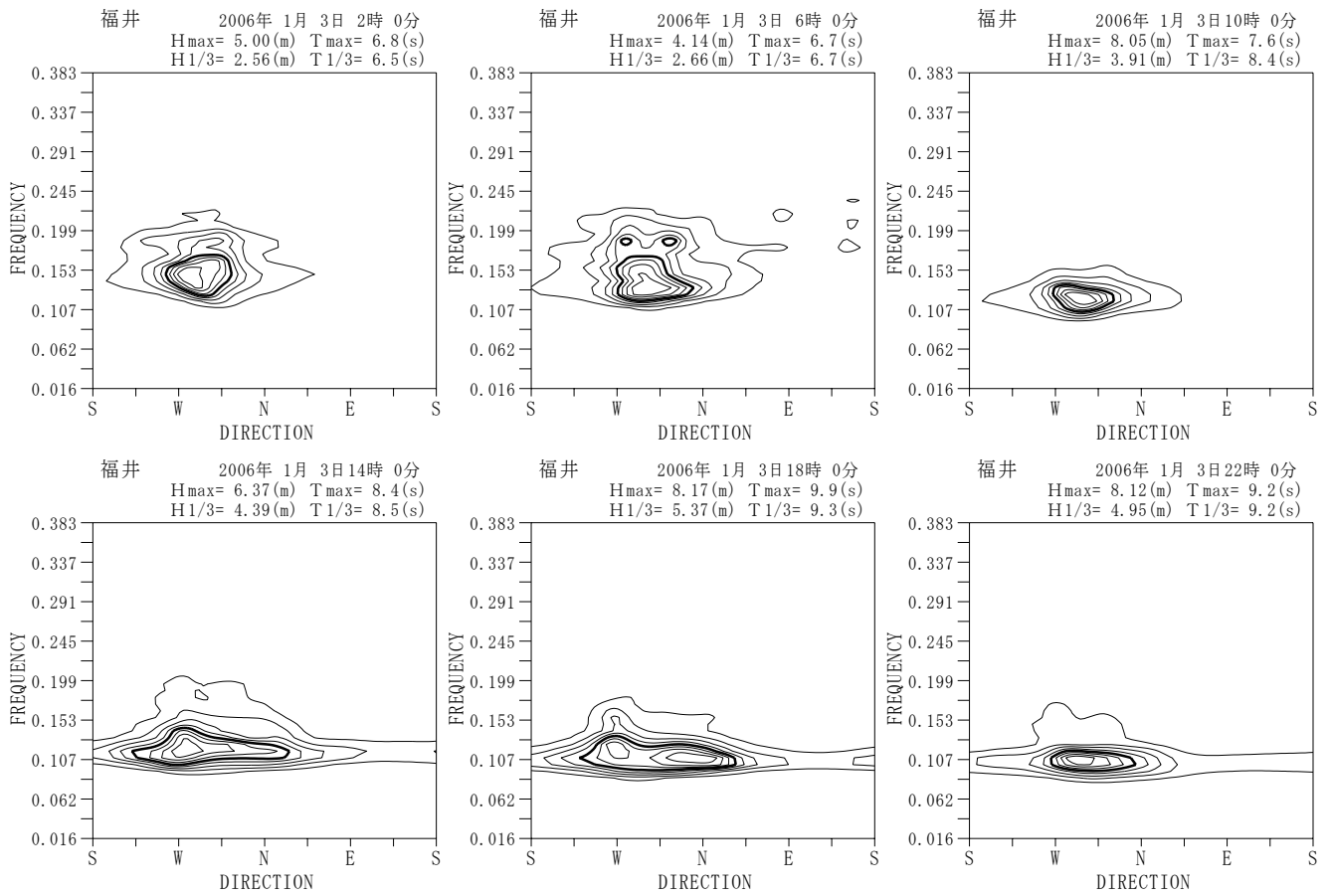
付図-A. 5. 14 福井 代表的な高波期間中の方向スペクトル
