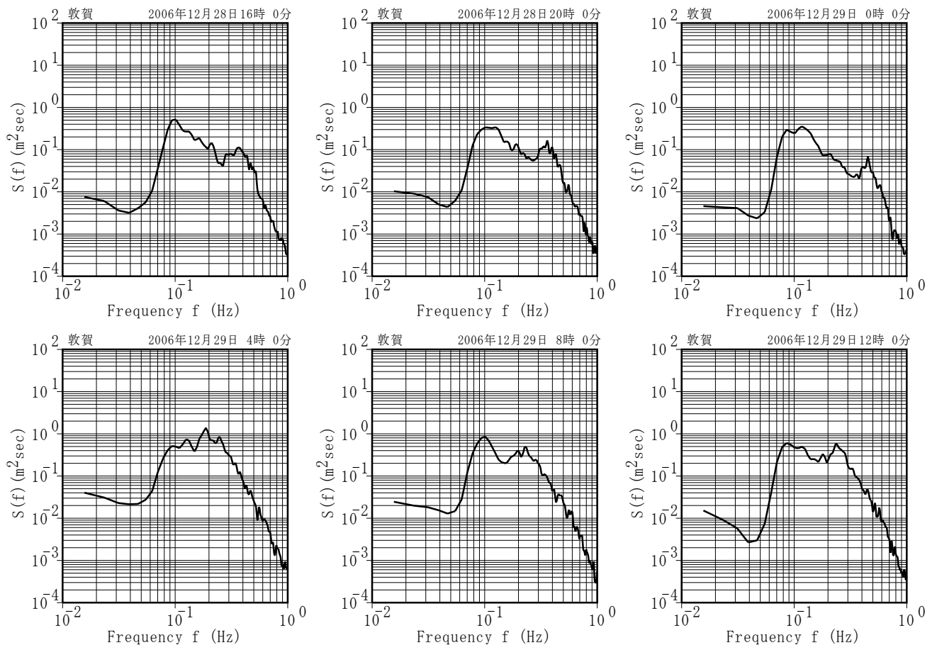
付図-A.5.15 敦賀 代表的な高波期間中のスペクトル
