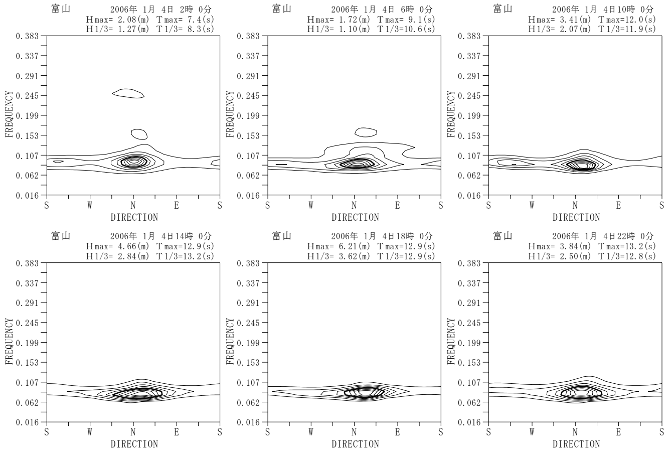
付図-A. 5. 10 富山 代表的な高波期間中の方向スペクトル
