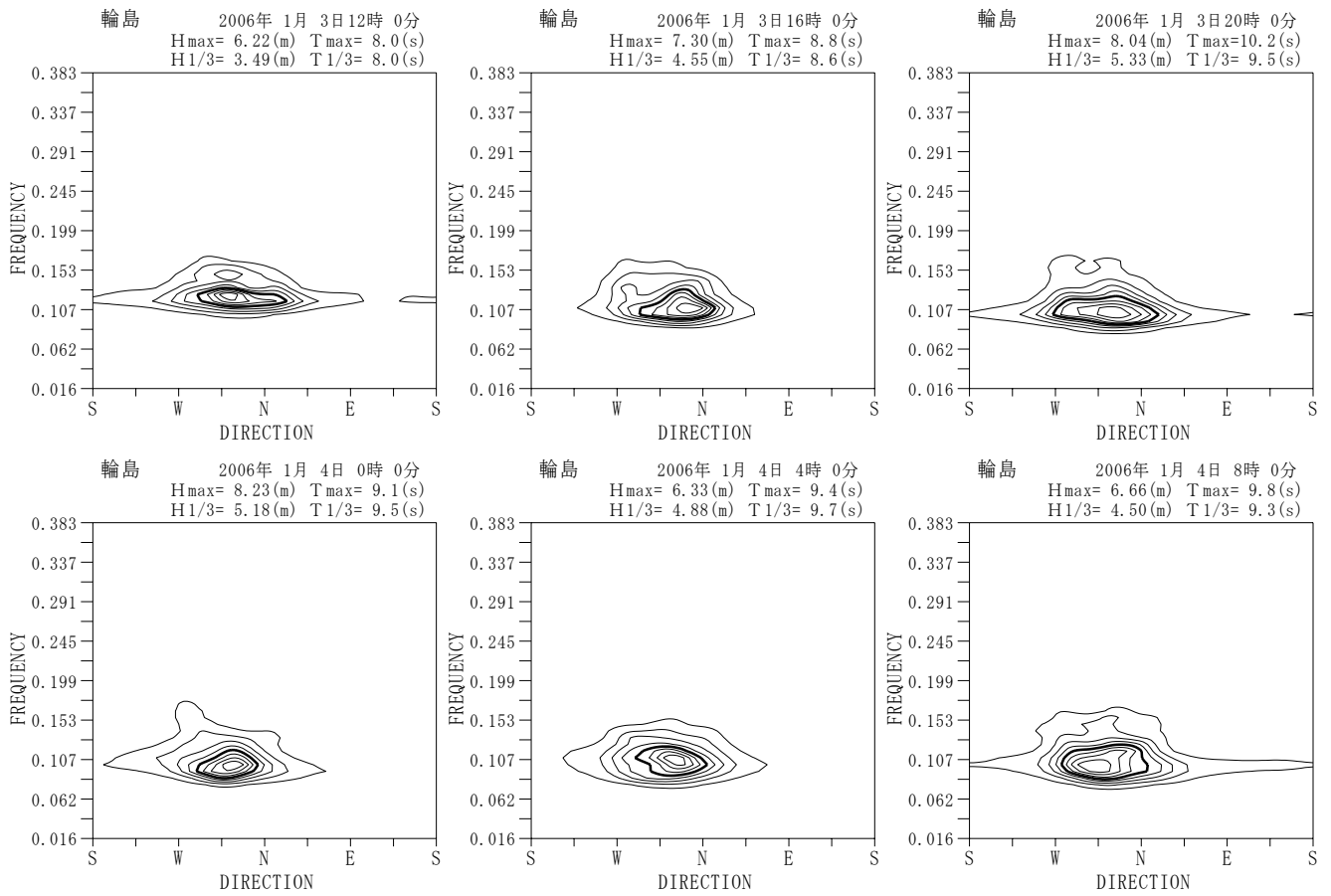
付図-A. 5. 12 輪島 代表的な高波期間中の方向スペクトル
