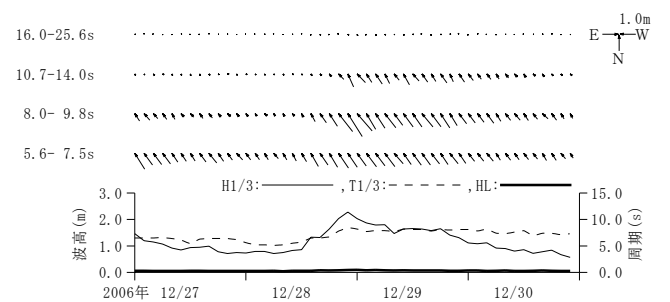
付図-A.3.60 平良沖 周期帯別波浪特性の経時変化(高波期間中)
