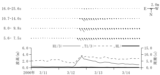
付図-A.3.60 平良沖 周期帯別波浪特性の経時変化(高波期間中)
