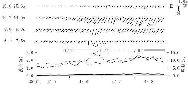
付図-A.3.27 紋別(南) 周期帯別波浪特性の経時変化(高波期間中)
