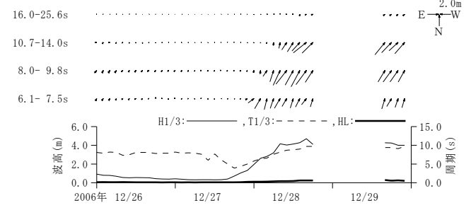
付図-A.3.27 紋別(南) 周期帯別波浪特性の経時変化(高波期間中)
