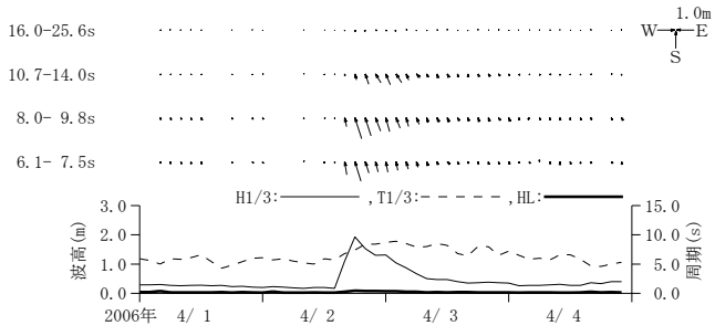
付図-A. 3. 45 清水 周期帯別波浪特性の経時変化(高波期間中)
