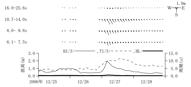
付図-A. 3. 45 清水 周期帯別波浪特性の経時変化(高波期間中)
