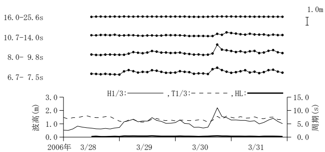
付図-A.3.44 下田 周期帯別波浪特性の経時変化(高波期間中)
