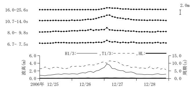
付図-A.3.44 下田 周期帯別波浪特性の経時変化(高波期間中)
