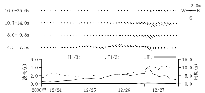
付図-A. 3. 46 御前崎 周期帯別波浪特性の経時変化(高波期間中)
