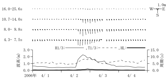
付図-A. 3. 46 御前崎 周期帯別波浪特性の経時変化(高波期間中)
