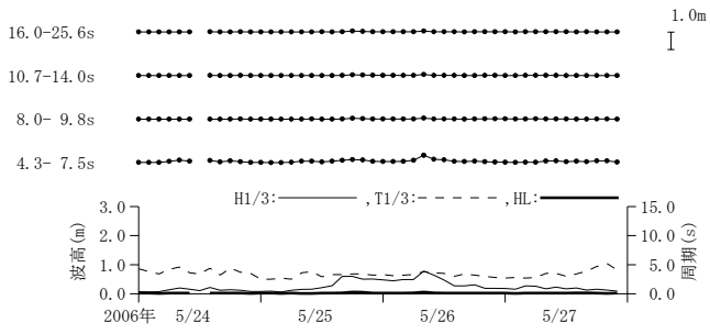
付図-A. 3. 58 鹿兒島 周期帯別波浪特性の経時変化(高波期間中)
