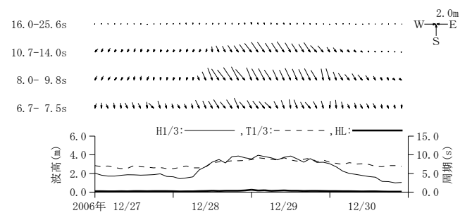
付図-A. 3. 25 名瀬 周期帯別波浪特性の経時変化(高波期間中)
