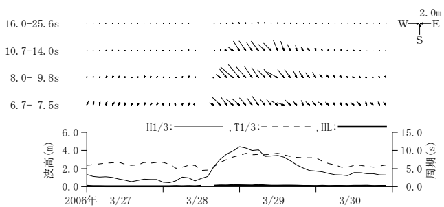
付図-A. 3. 25 名瀬 周期帯別波浪特性の経時変化(高波期間中)
