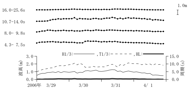
付図-A.3.17 柴山(港内) 周期帯別波浪特性の経時変化(高波期間中)
