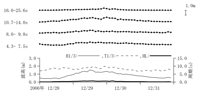
付図-A.3.17 柴山(港内) 周期帯別波浪特性の経時変化(高波期間中)
