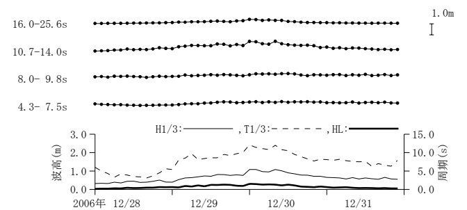
付図-A. 3. 19 境港 周期帯別波浪特性の経時変化(高波期間中)
