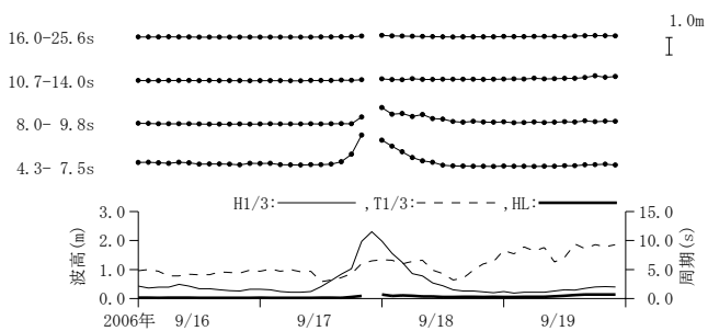
付図-A. 3. 19 境港 周期帯別波浪特性の経時変化(高波期間中)
