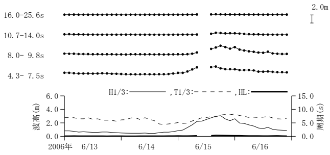
付図-A. 3. 53 高知 周期帯別波浪特性の経時変化(高波期間中)
