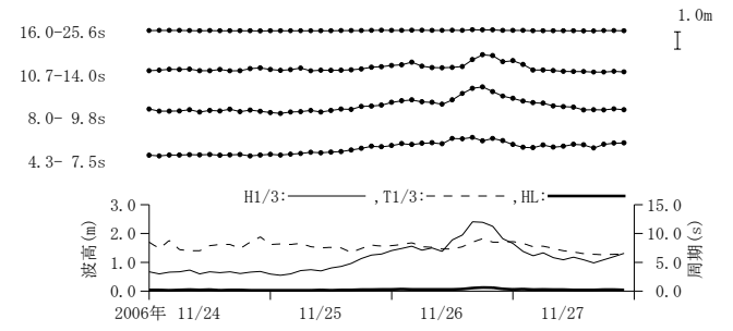
付図-A. 3. 53 高知 周期帯別波浪特性の経時変化(高波期間中)
