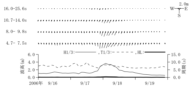
付図-A. 3. 52 室津 周期帯別波浪特性の経時変化(高波期間中)
