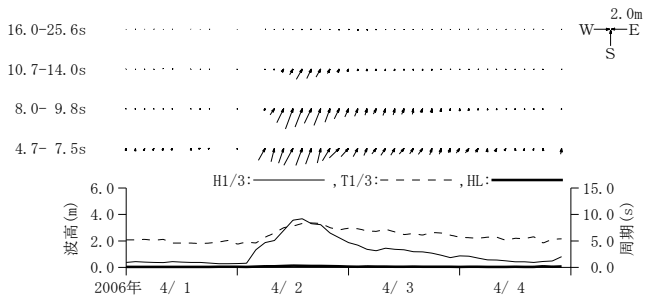
付図-A. 3. 52 室津 周期帯別波浪特性の経時変化(高波期間中)
