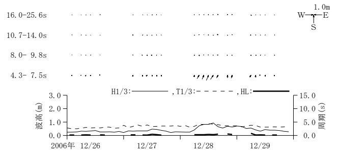
付図-A.3.49 神戸 周期帯別波浪特性の経時変化(高波期間中)
