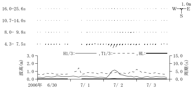
付図-A.3.49 神戸 周期帯別波浪特性の経時変化(高波期間中)
