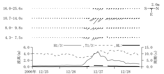
付図-A. 3.35 石巻 周期帯別波浪特性の経時変化(高波期間中)
