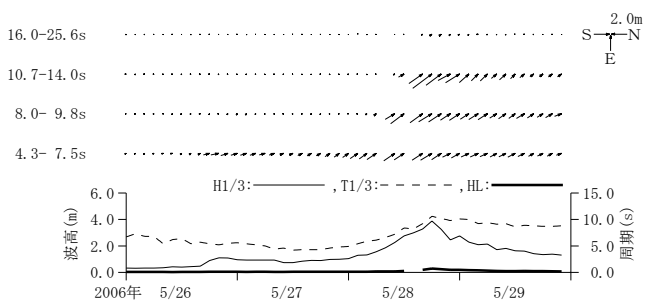
付図-A. 3.35 石巻 周期帯別波浪特性の経時変化(高波期間中)
