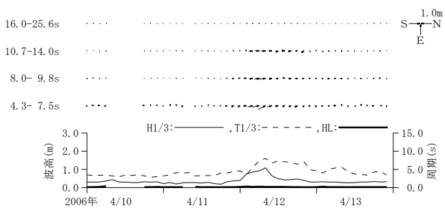
付図-A.3.41 第二海堡 周期帯別波浪特性の経時変化(高波期間中)
