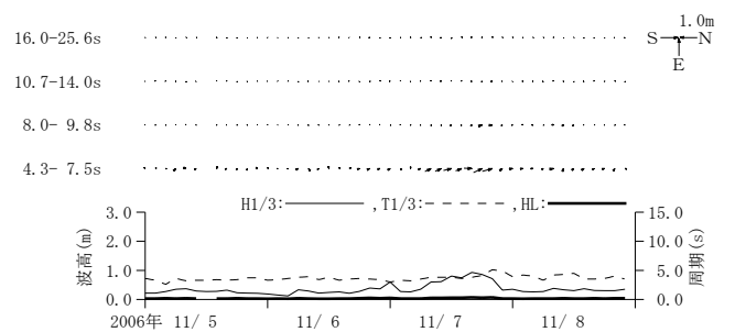
付図-A.3.41 第二海堡 周期帯別波浪特性の経時変化(高波期間中)
