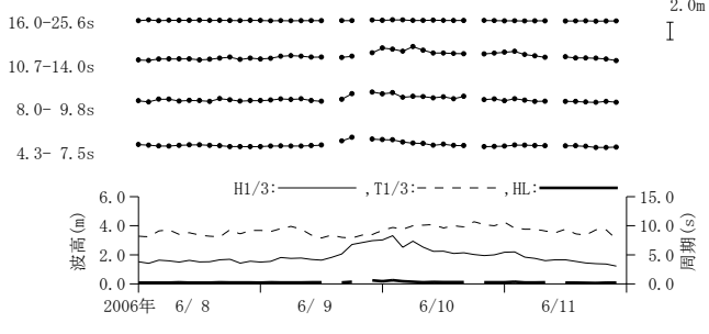
付図-A. 3.37 相馬 周期帯別波浪特性の経時変化(高波期間中)
