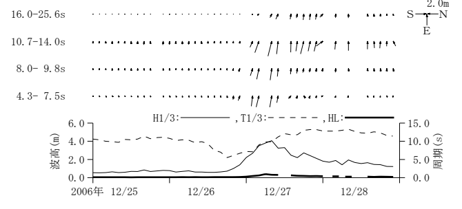
付図-A. 3.37 相馬 周期帯別波浪特性の経時変化(高波期間中)
