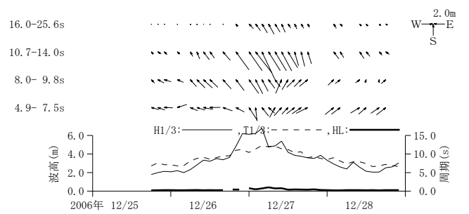
付図-A. 3. 43 波浮 周期帯別波浪特性の経時変化(高波期間中)
