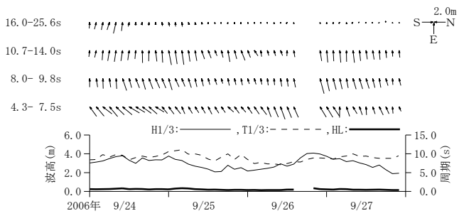
付図-A. 3. 40 鹿島 周期帯別波浪特性の経時変化(高波期間中)
