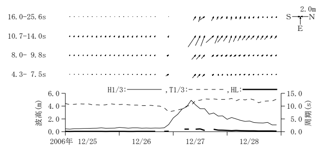
付図-A. 3.36 仙台新港 周期帯別波浪特性の経時変化(高波期間中)
