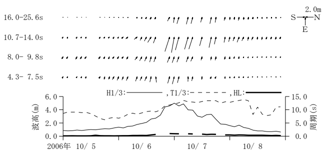
付図-A. 3.36 仙台新港 周期帯別波浪特性の経時変化(高波期間中)
