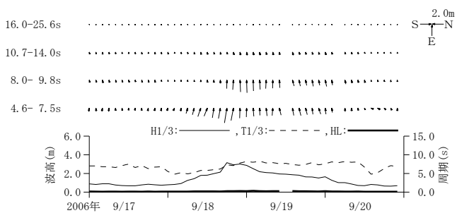
付図-A. 3. 32 八戸 周期帯別波浪特性の経時変化(高波期間中)
