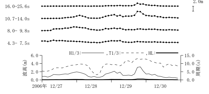
付図-A.3.10 富山 周期帯別波浪特性の経時変化(高波期間中)
