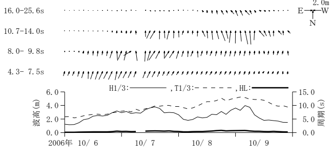
付図-A.3.10 富山 周期帯別波浪特性の経時変化(高波期間中)
