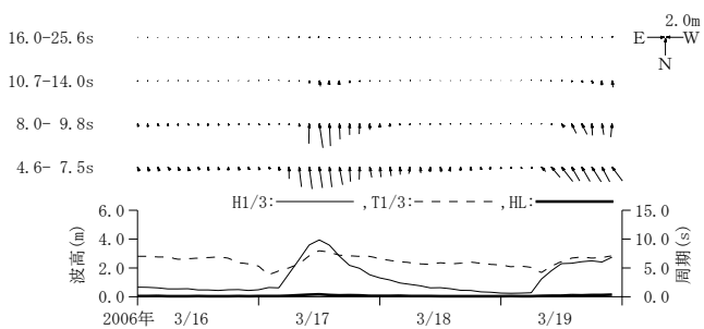
付図-A.3.8 新潟沖 周期帯別波浪特性の経時変化(高波期間中)
