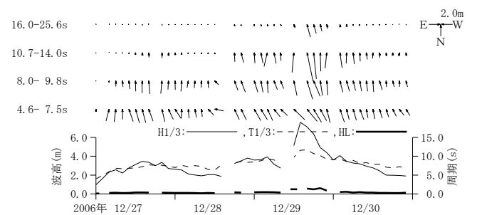
付図-A.3.8 新潟沖 周期帯別波浪特性の経時変化(高波期間中)
