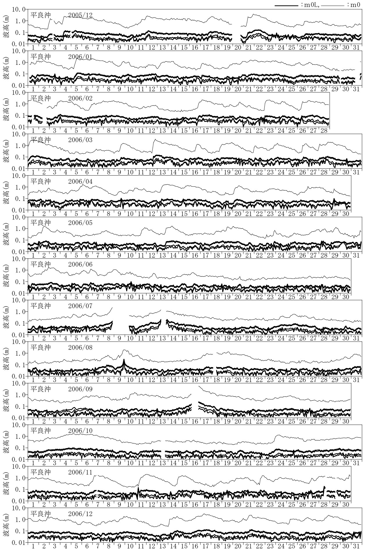
付図-C.1.60 長周期波高の経時変化図 (平良沖)
