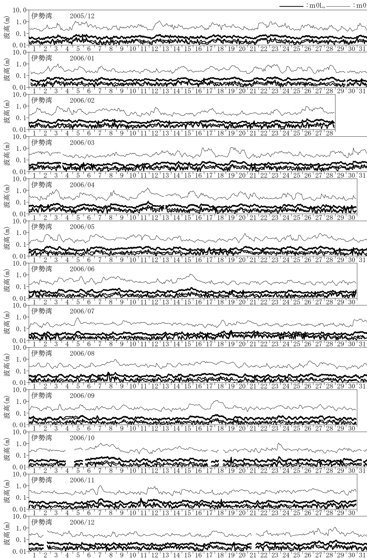
付図-C.1.47 長周期波高の経時変化図 (伊勢湾)
