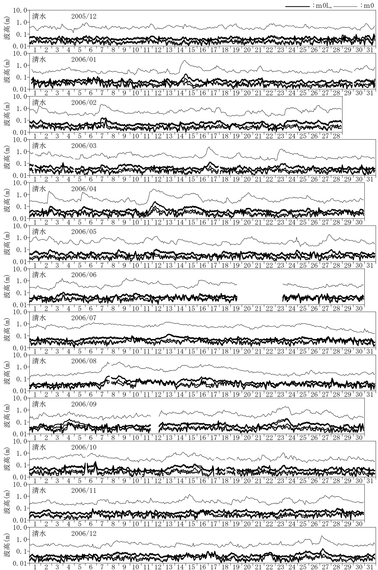
付図-C. 1.45 長周期波高の経時変化図 (清水)
