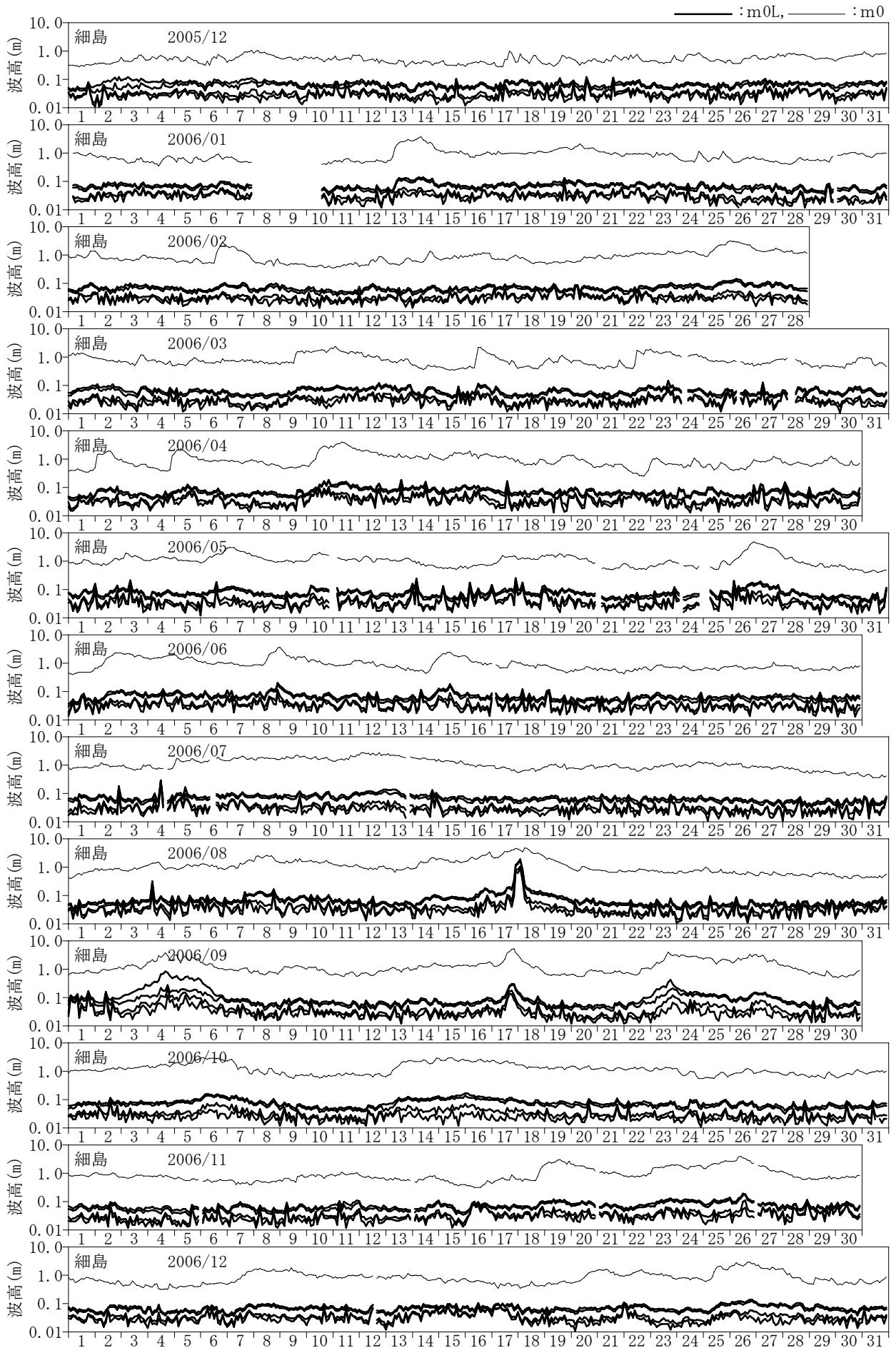
付図-C.1.56 長周期波高の経時変化図 (細島)
