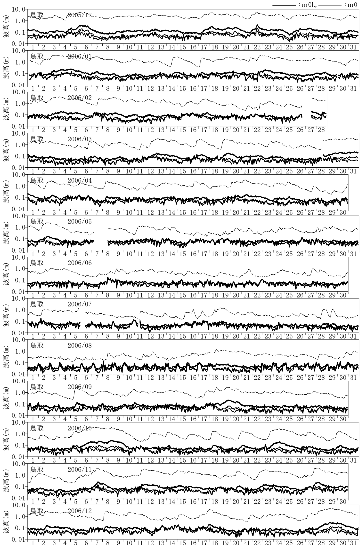
付図-C.1.18 長周期波高の経時変化図 (鳥取)
